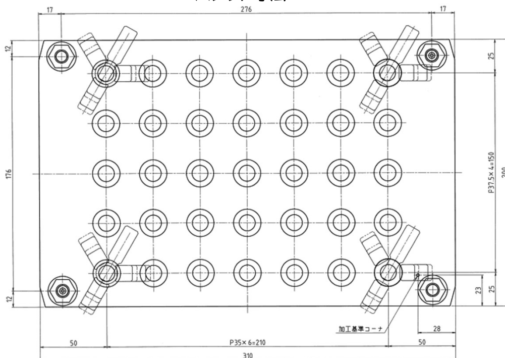
パレット寸法
